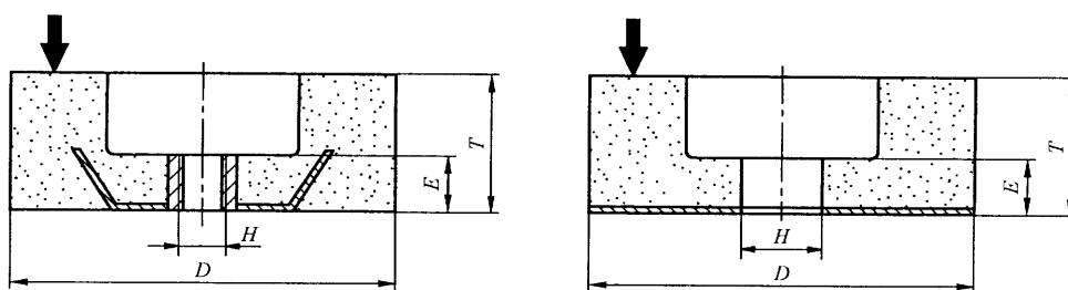
图 2 6 型 有插入的紧固衬套或完全的金属背垫
