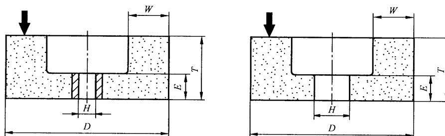
图 1 6 型 无插入的紧固衬套或完全的金属背垫
