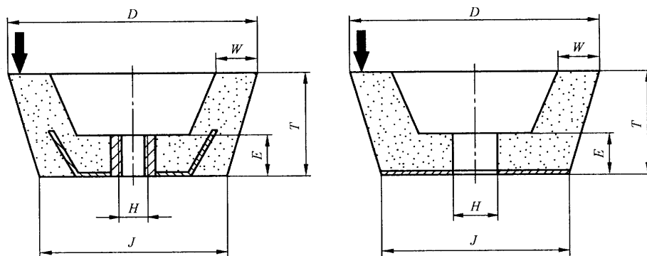
图 4 11 型 有插入的紧固衬套或完全的金属背垫
