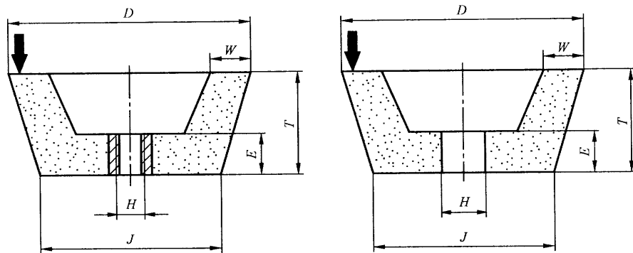
图 3 11 型 无插入的紧固衬套或完全的金属背垫
